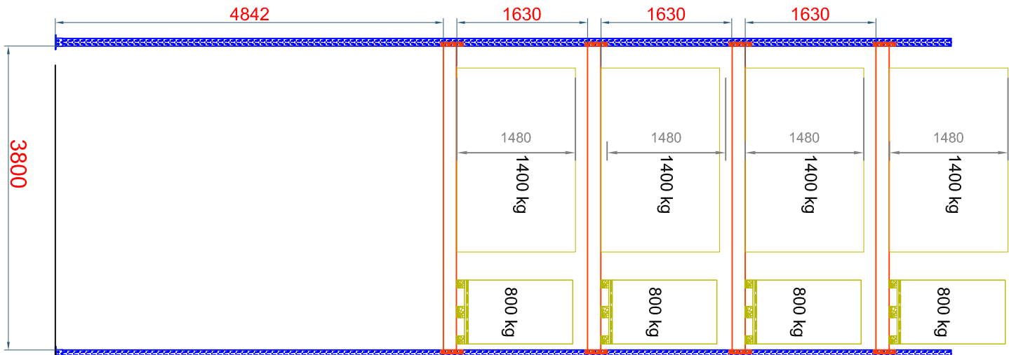
GAB 4M3P PRZEJAZD
